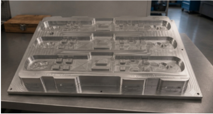
Moule de thermoformage pour supports électroniques
