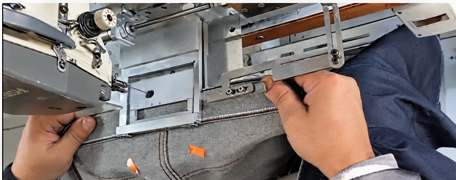
Dispositif de pose d'étiquettes
