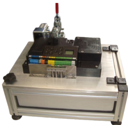
Machines de dégrappage des cartes électronique
