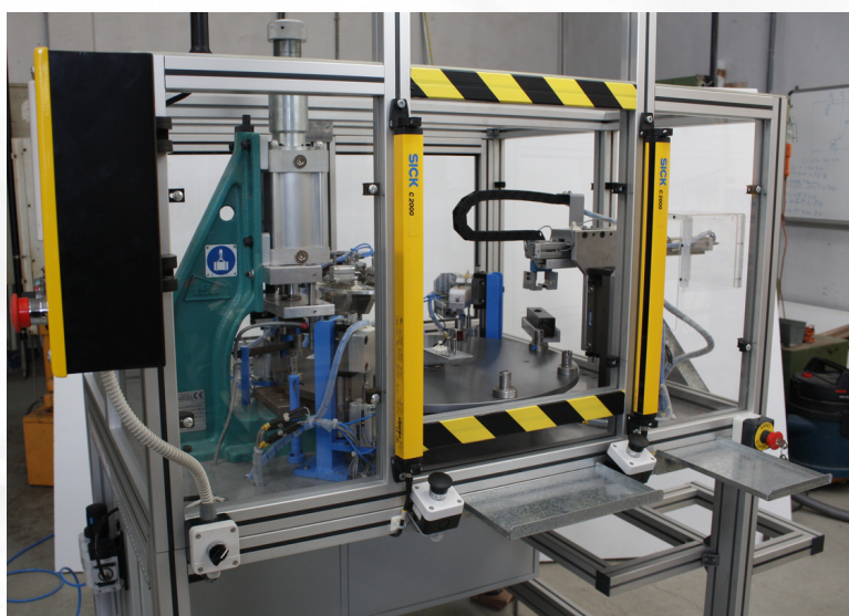
Machines d'assemblage allume Cigare
