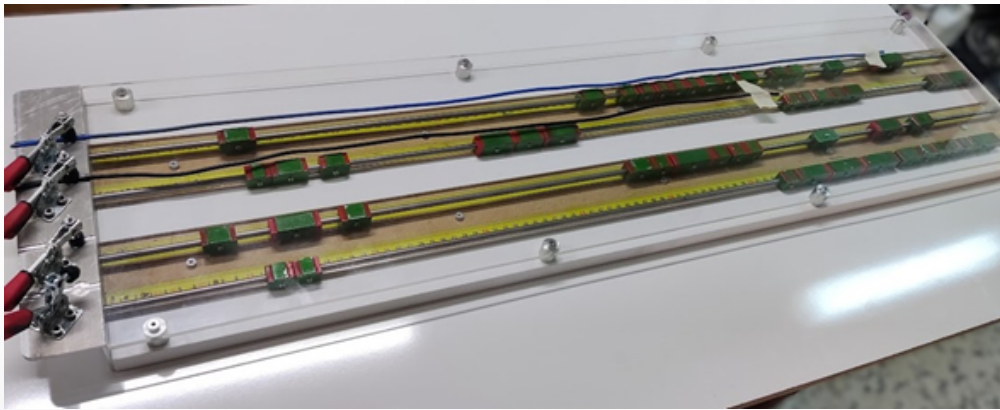
Gabarits de contrôle dimensionnelles
