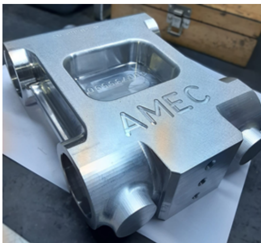
Porte bielle du système mécanique Pantographe
